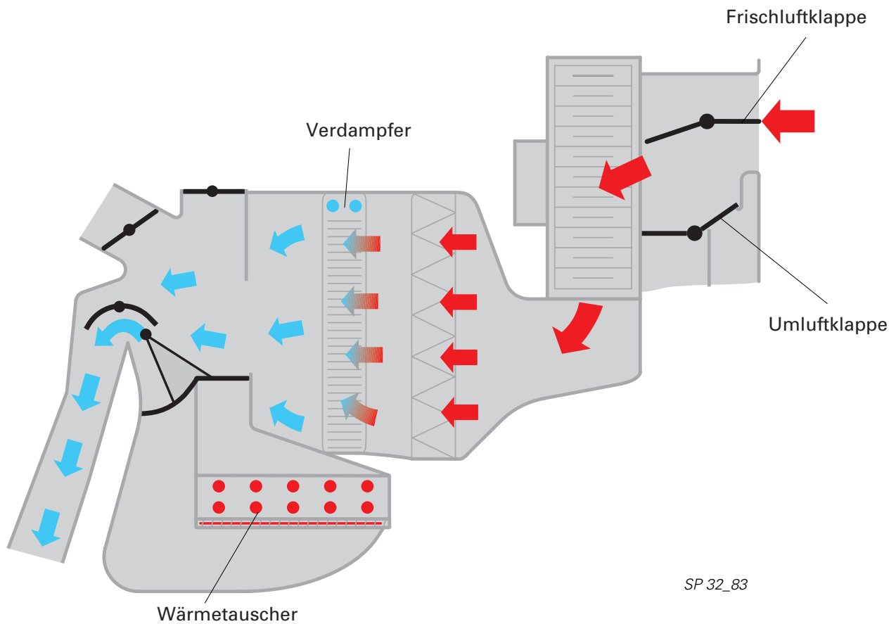
Luftführung bei Stellung Frischluft und gekühlte Innenluftzuführung
